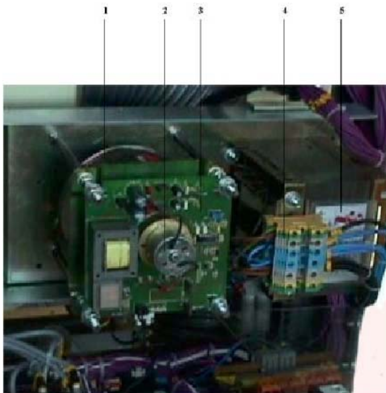
FIG. 9 - DESCRIZIONE STABILIZZATORE DI TENSIONE
