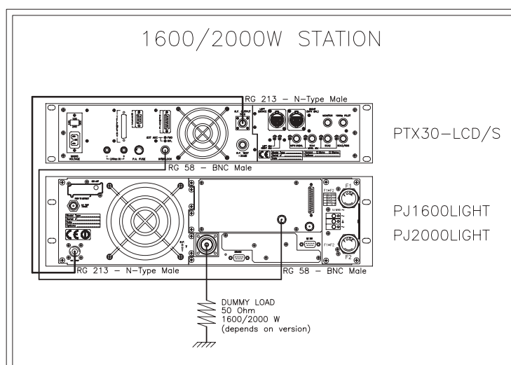
Figura 5.1: collegamento con l'amplificatore
