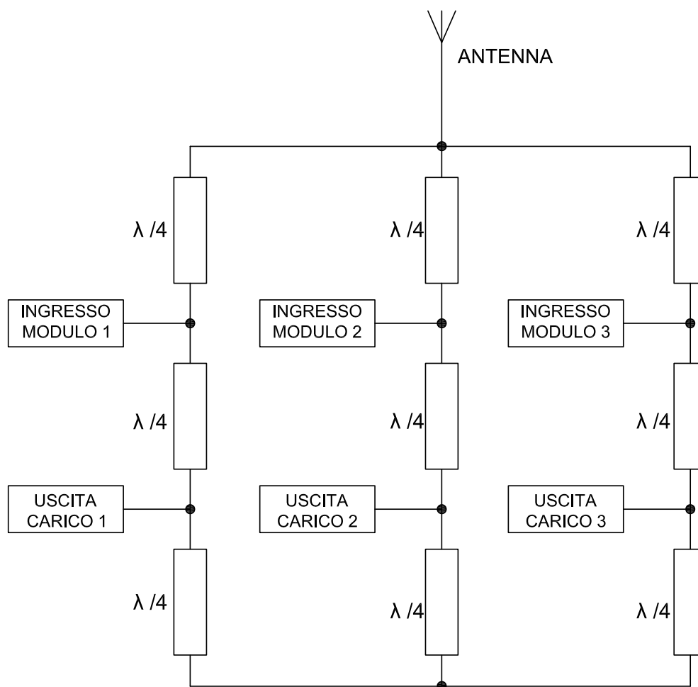
Vista interna
