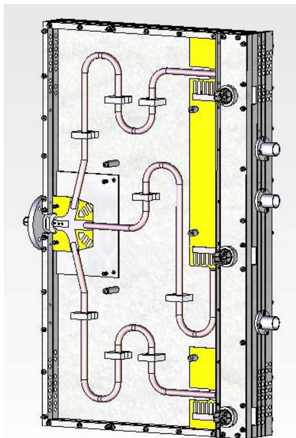
Vista interna
